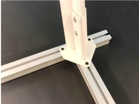
Plattenrahmen Alu natur eloxiert, Fusspositionierung 90°
