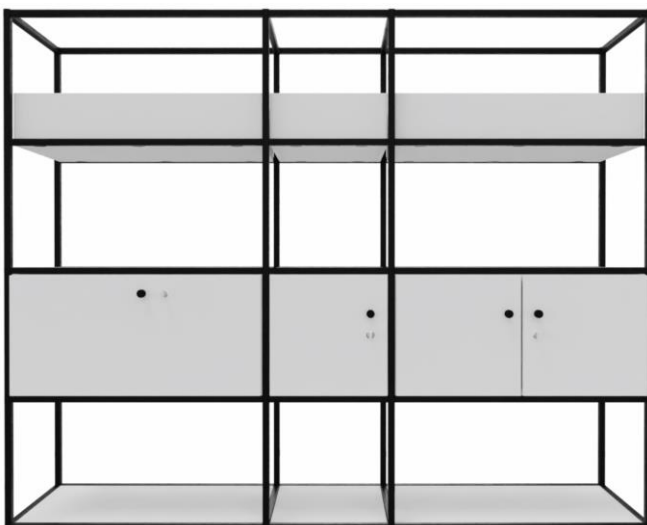
2000 x 400 x 1590 mm 6 x offen / 1 x Klappe / 1 x Flügeltüre / 1 x Doppelflügeltüre / 3 x Pflanzenmodul
