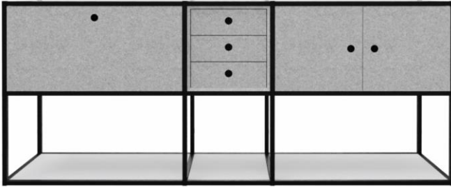
2000 x 400 x 810 mm 3 x offen / 1 x Klappe / 1 x 3 Schubladen / 1 x Flügeltüren Korpusse Ausführung PET A
